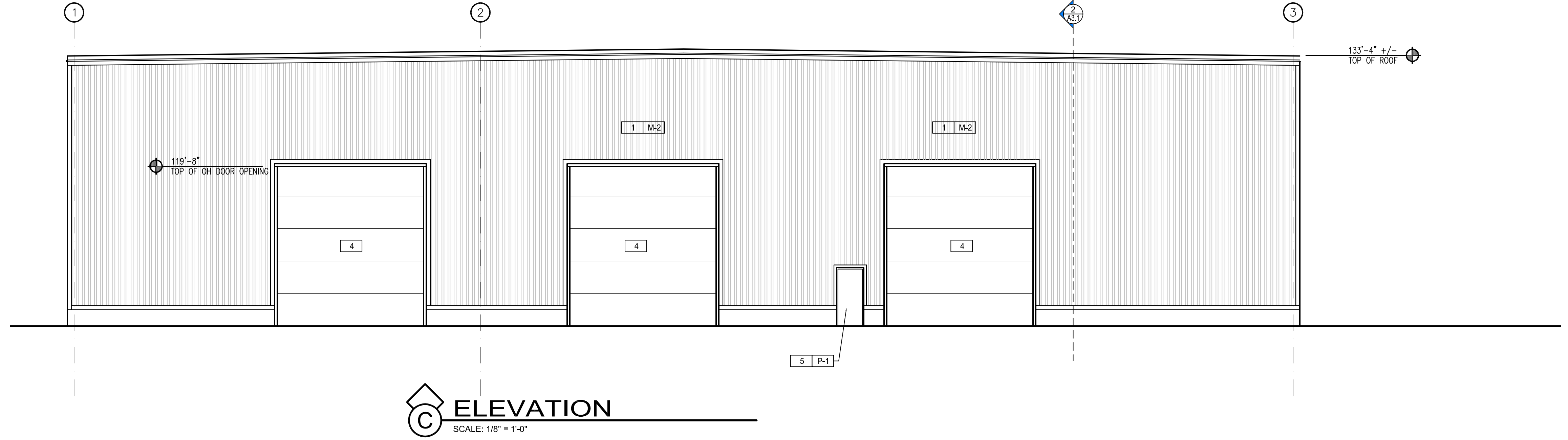
B ELEVATION SCALE: 1/8" = 1'-0"
