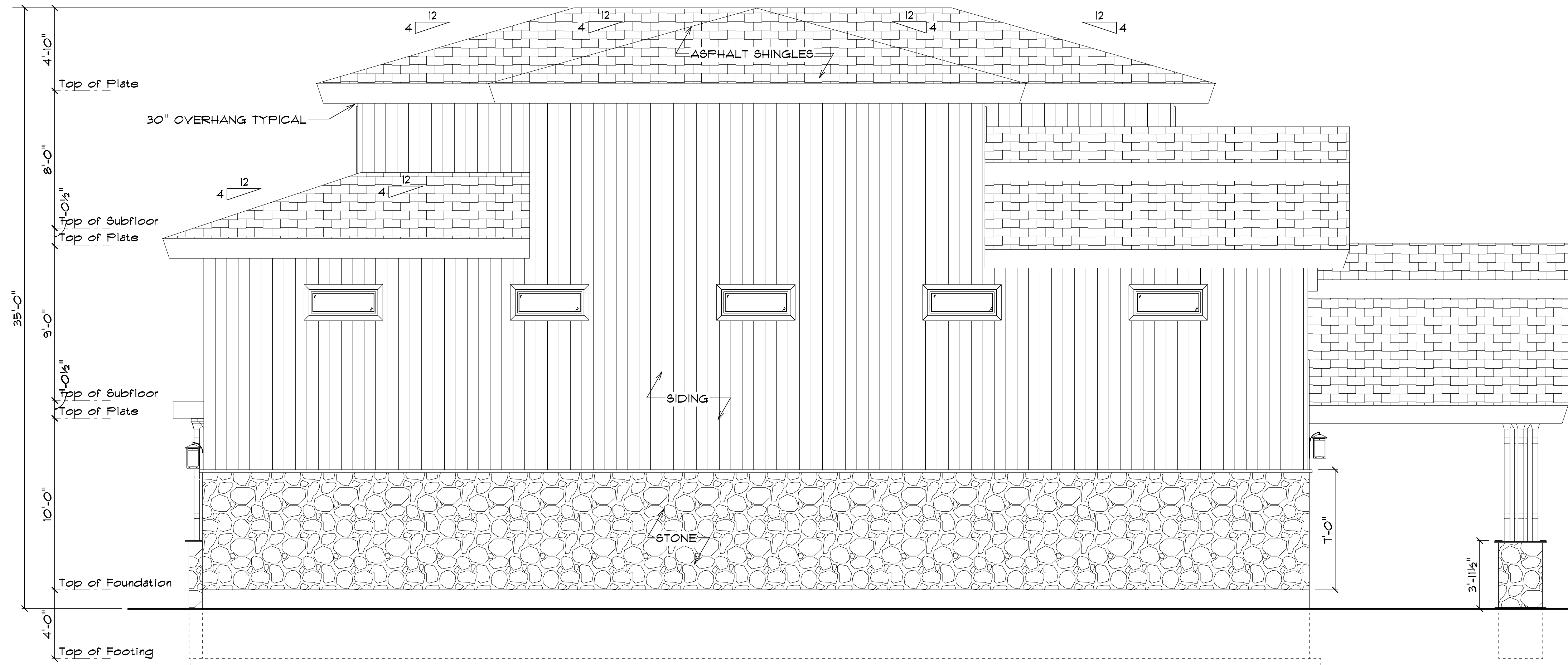
Left SCALE: 1/4" = 1'-0"
