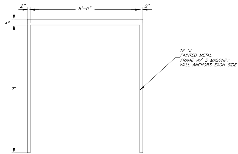
FRAME TYPE B SCALE: NONE
