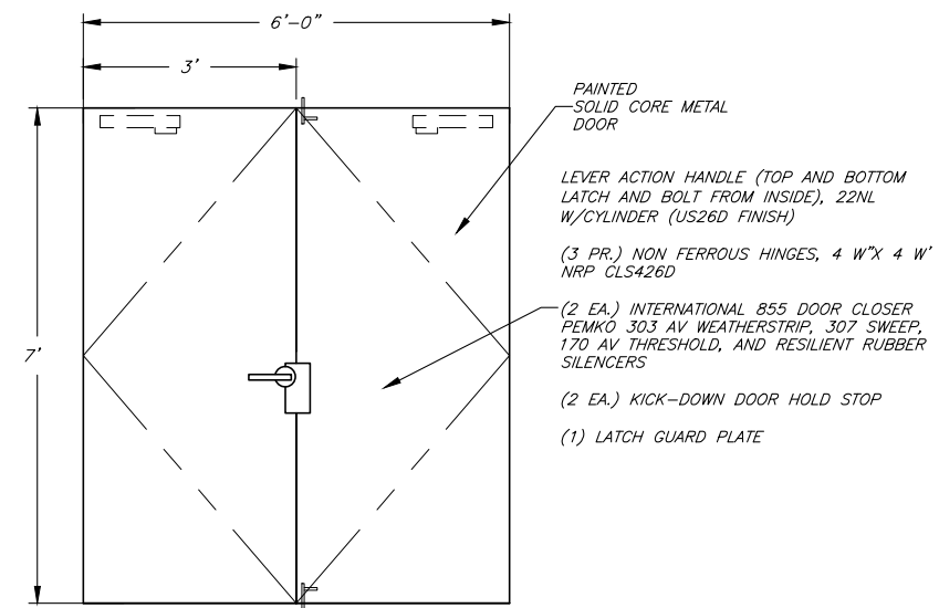
DOOR TYPE B SCALE: NONE
