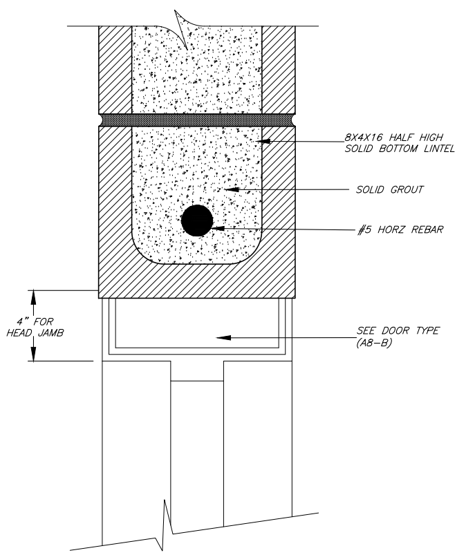
LINTEL DETAIL 4 SCALE: NONE
