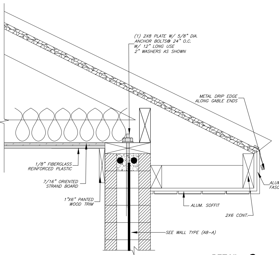
DETAIL 2 SCALE: NONE
