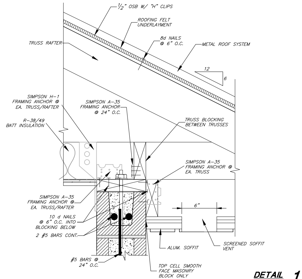
DETAIL 1 SCALE: NONE
