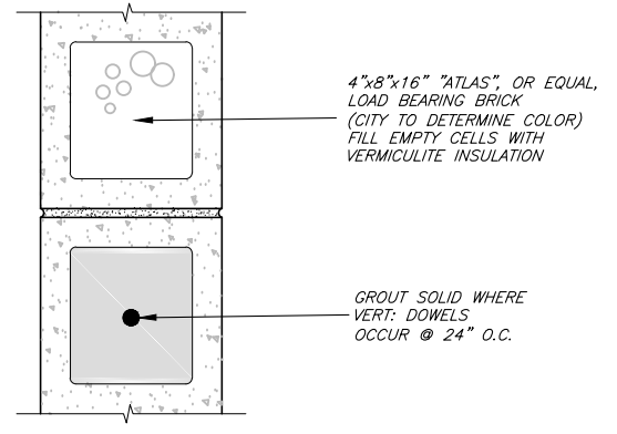
WALL TYPE A SCALE: NONE
