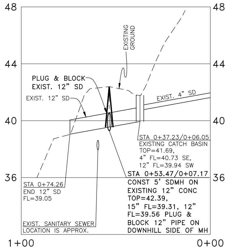
SECTION 'A'
