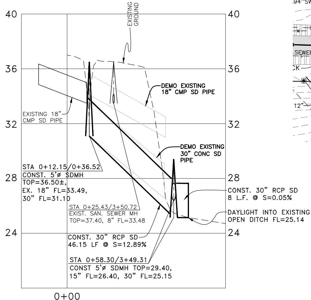
SECTION 'B'
