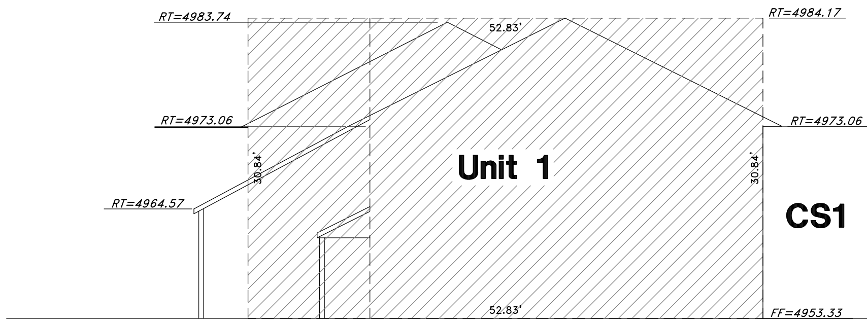
Section A-A
