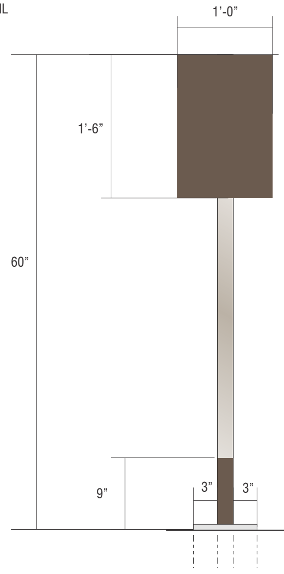
BACK VIEW SCALE: 1"=1'-0"
