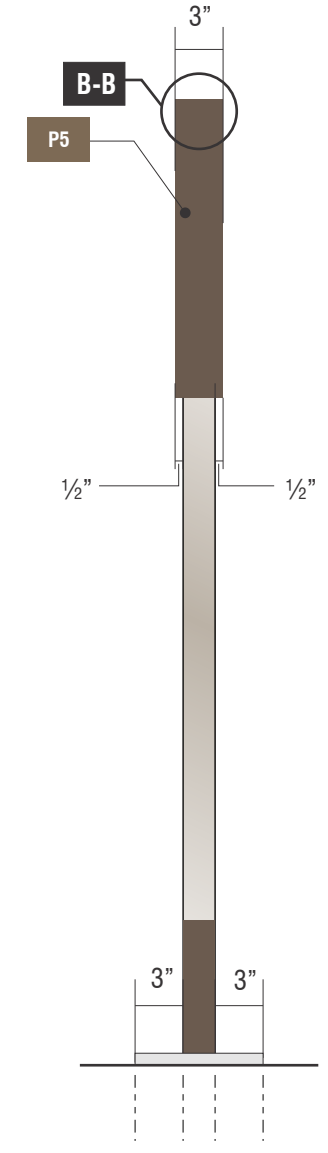
END VIEW SCALE: 1"=1'-0"
