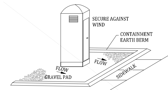
M PORTABLE TOILET -- SCALE: NONE
