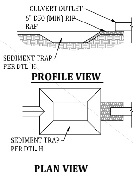
OUTLET PROTECTION SCALE: NONE
