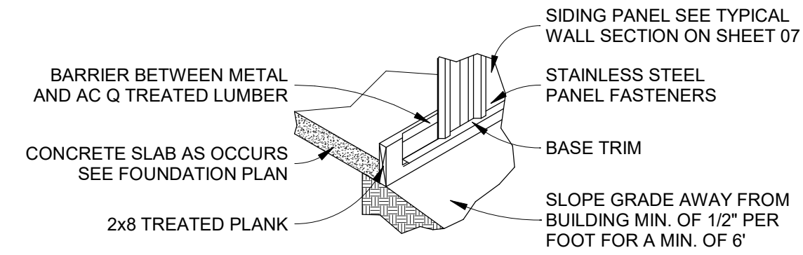
③ BASE GUARD FLASHING N.T.S.
