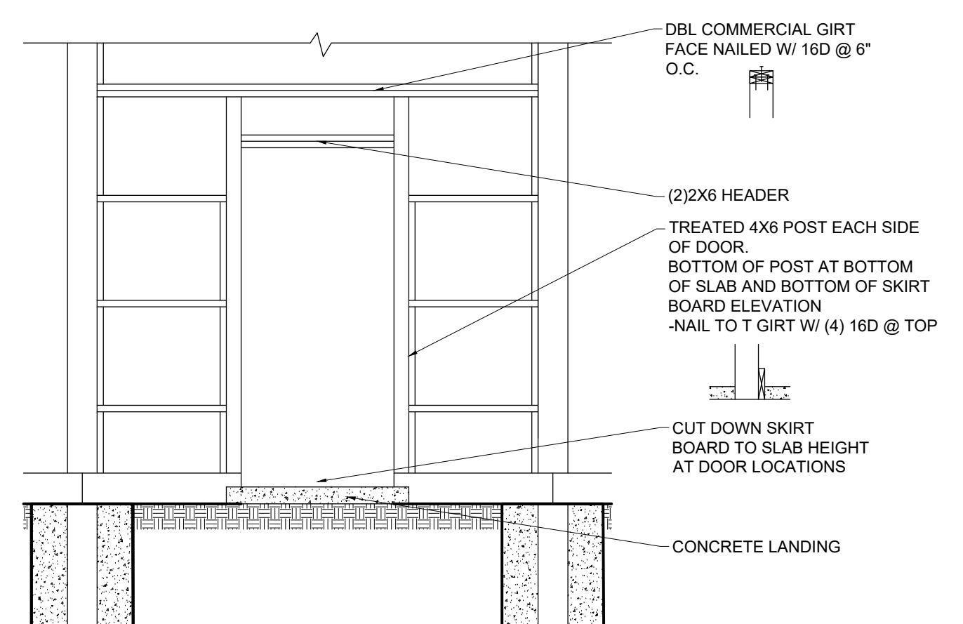
13 MAN DOOR FRAMING A8 NTS
