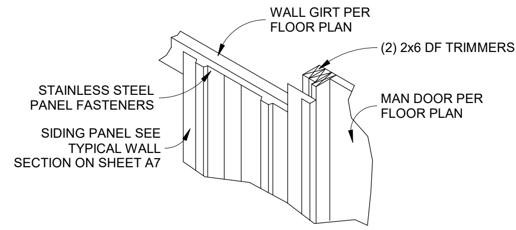
① MAN DOOR JAMB FLASHING N.T.S.
