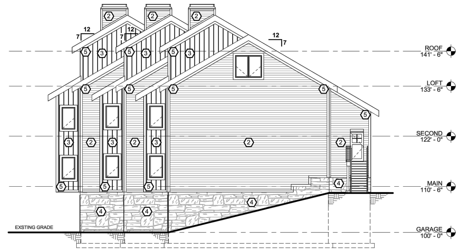
RIGHT ELEVATION
