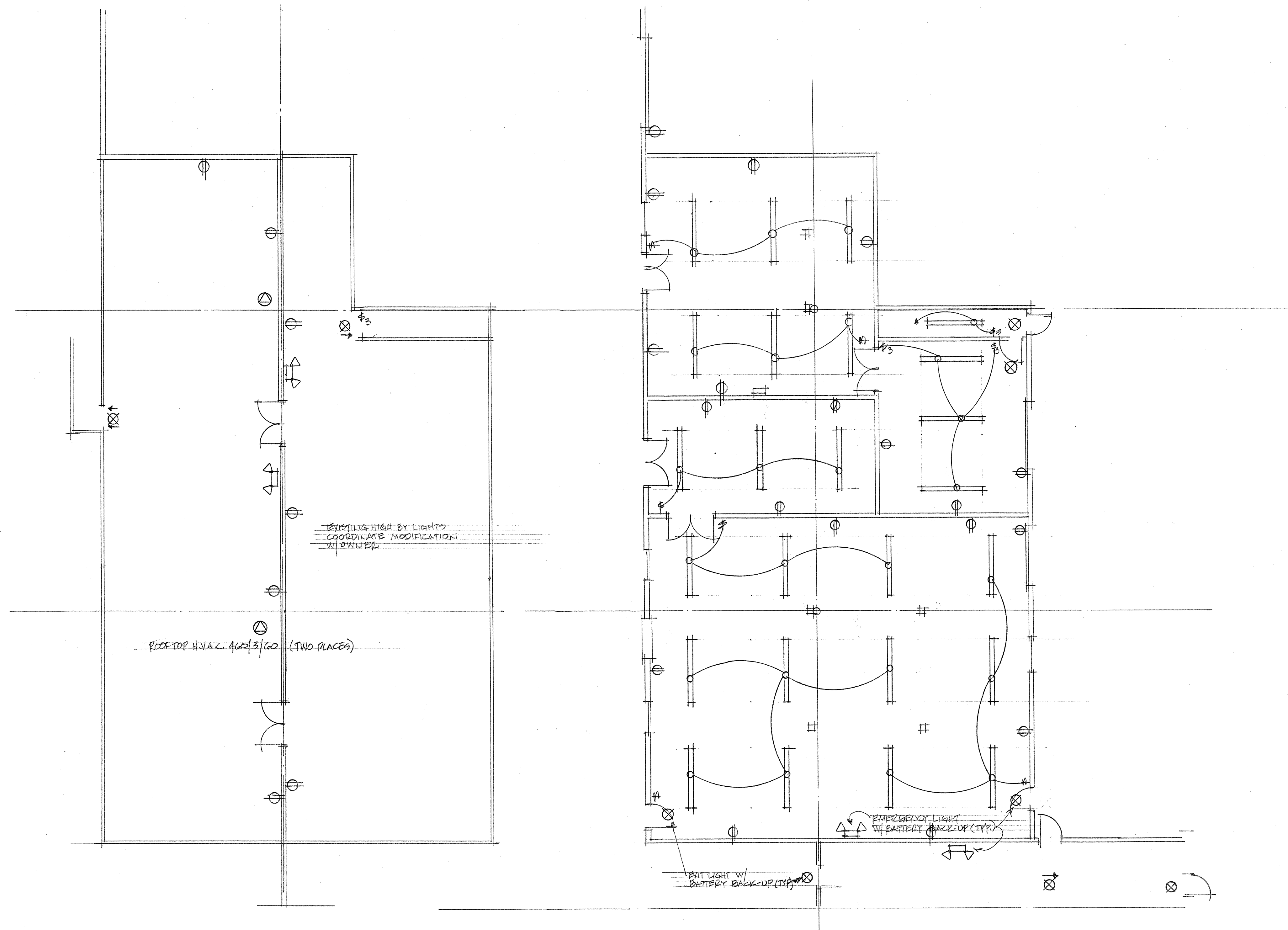
UPPER MEZ. ELECTRICAL PLAN SCALE: 1/8" = 1'-0"
