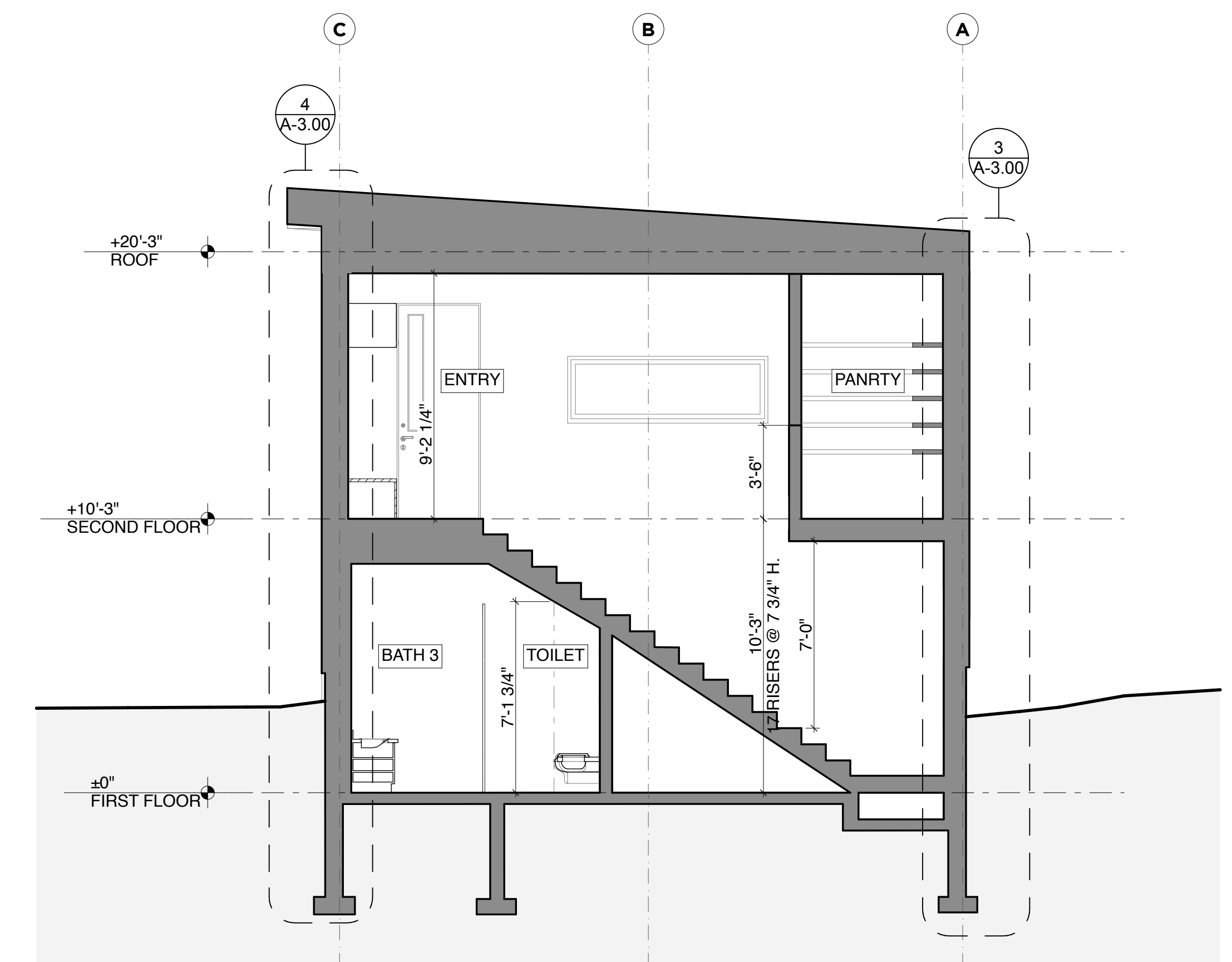
STAIR SECTION 2 SCALE: 1/4" = 1'-0"
