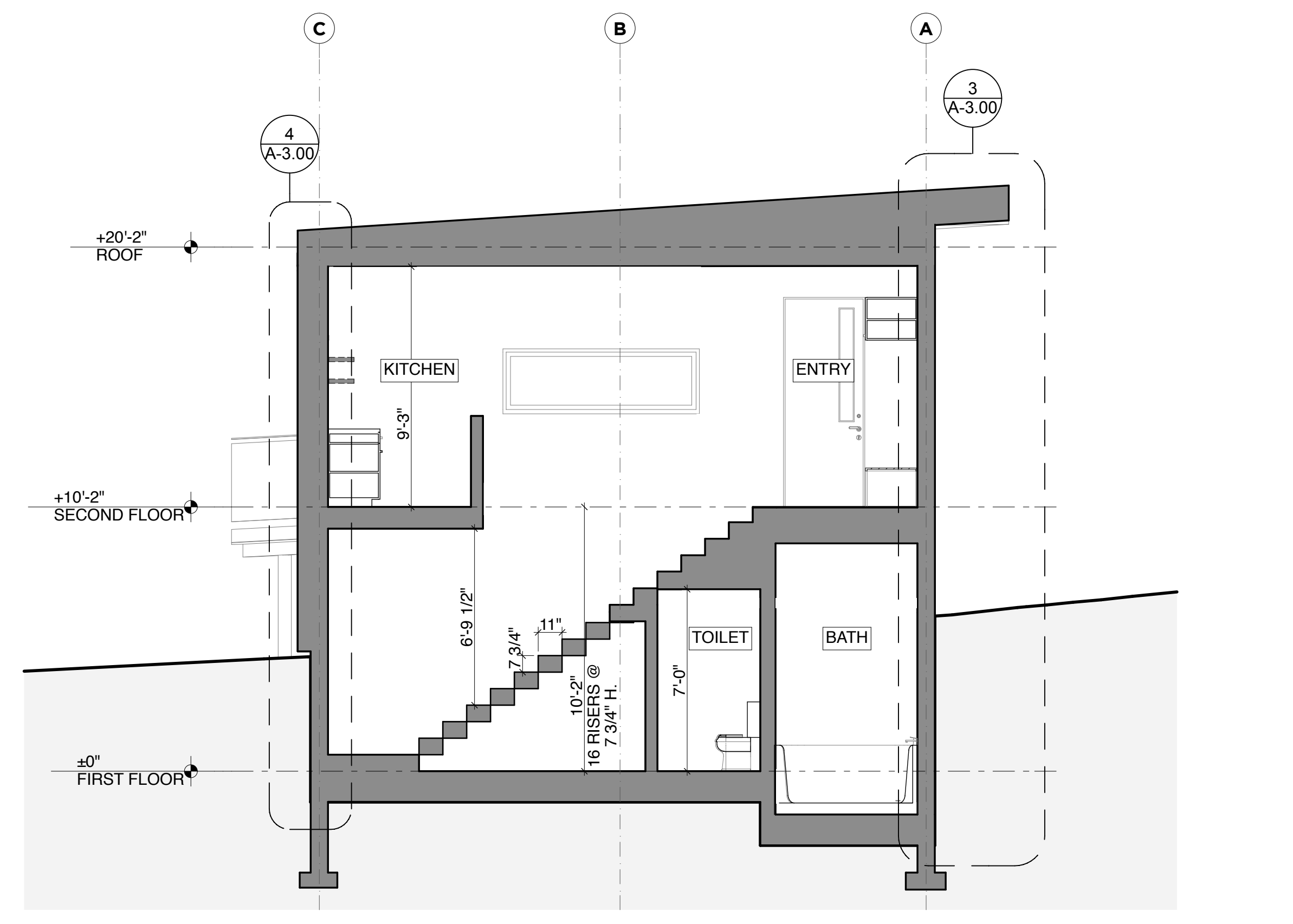
N-S SECTION SCALE: 1/4" = 1'-0" 2
