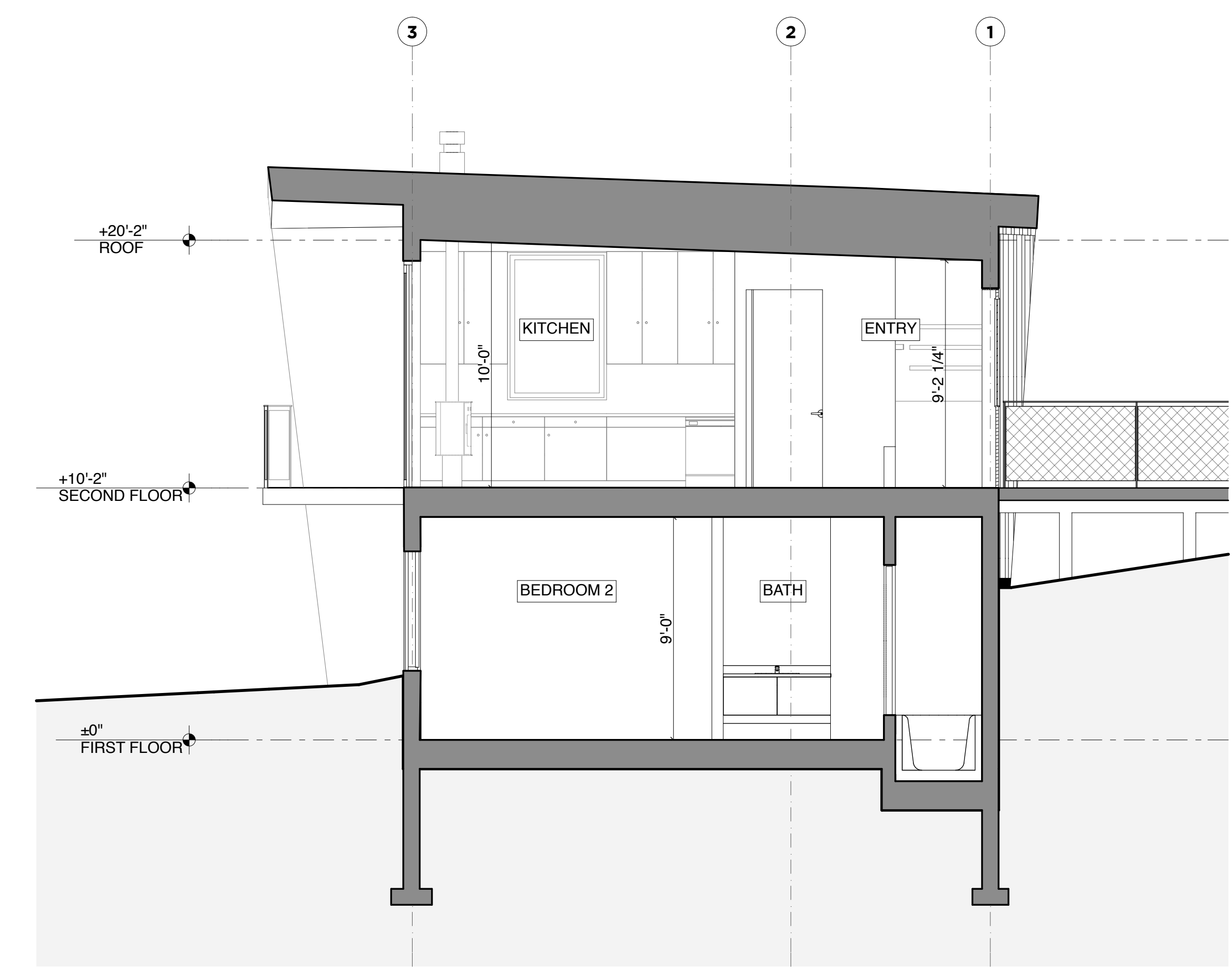
E-W SECTION SCALE: 1/4" = 1'-0" 1
