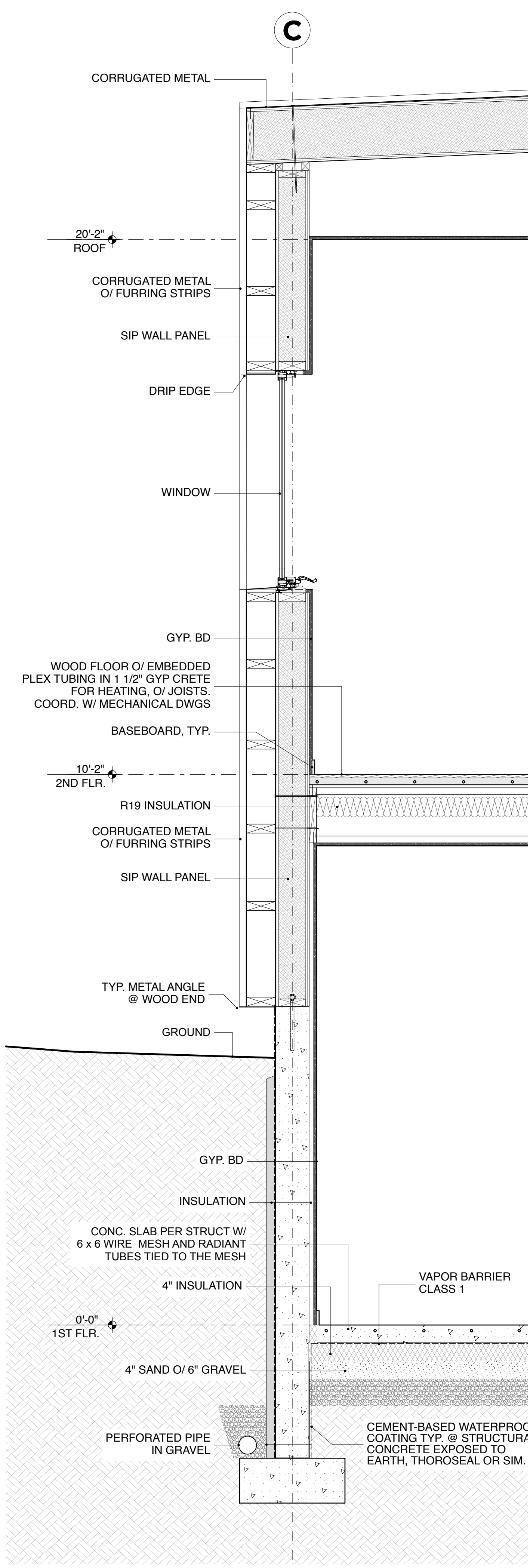
METAL WALL SECTION SCALE: 3/4" = 1'-0" 4
