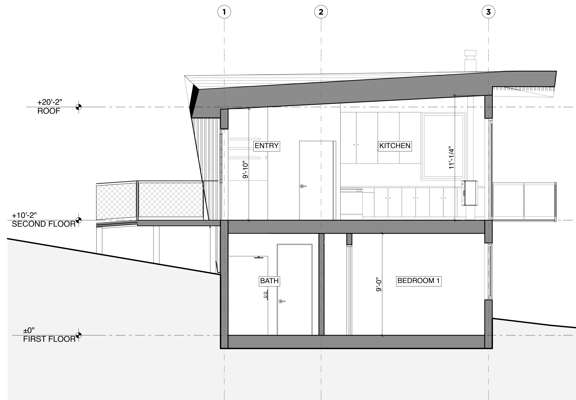
E-W SECTION SCALE: 1/4" = 1'-0"
