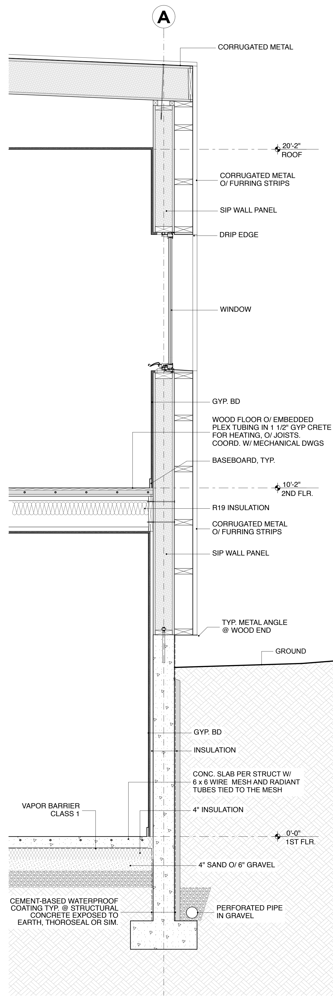
METAL WALL SECTION SCALE: 3/4" = 1'-0"
