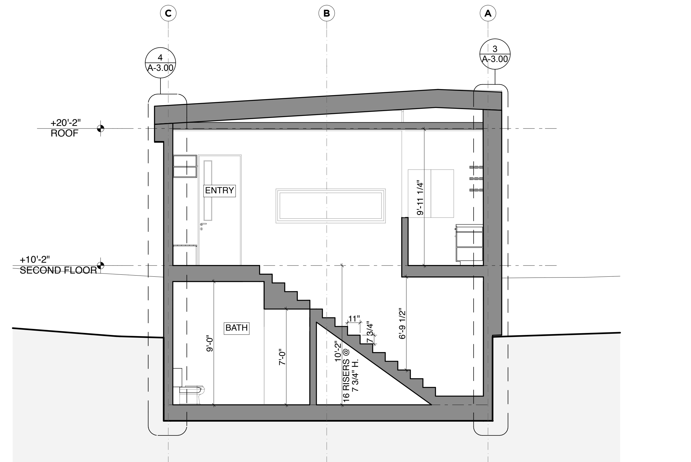
N-S SECTION SCALE: 1/4" = 1'-0"
