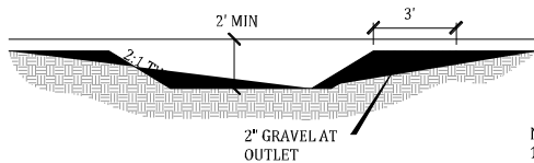
F -- ROCK CHECK DAM SCALE: NONE
