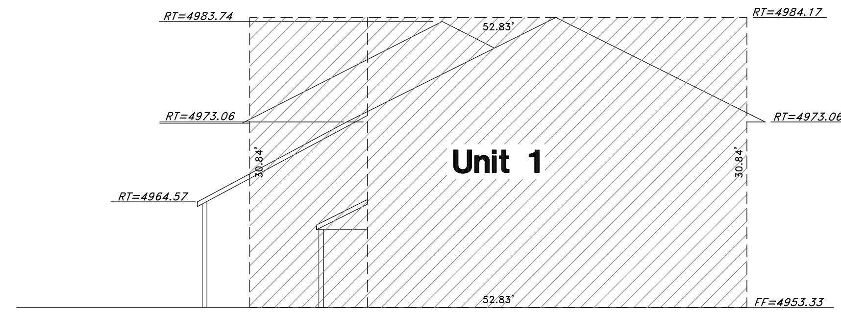
Section A-A
